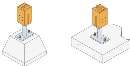
Fixation du PISB160G- K sur support rigide
